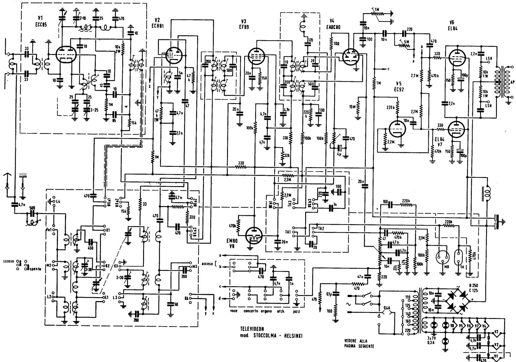
Schema elettrico del radiorecettore AM - FM, Televideon, mod. Stoccolma - Helsinki
